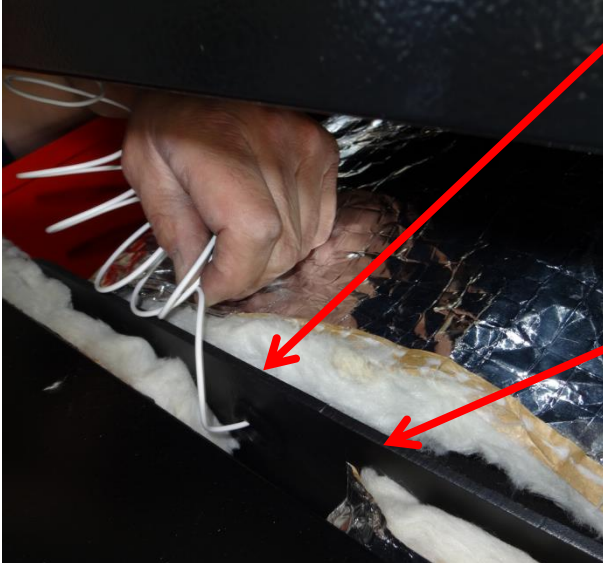
Sonda termometra ubacuje se u cev, do kraja cevi. Napomena: Obratiti pažnju da ne dođe do oštećenja kapilare i sonde termometra pri montaži.
