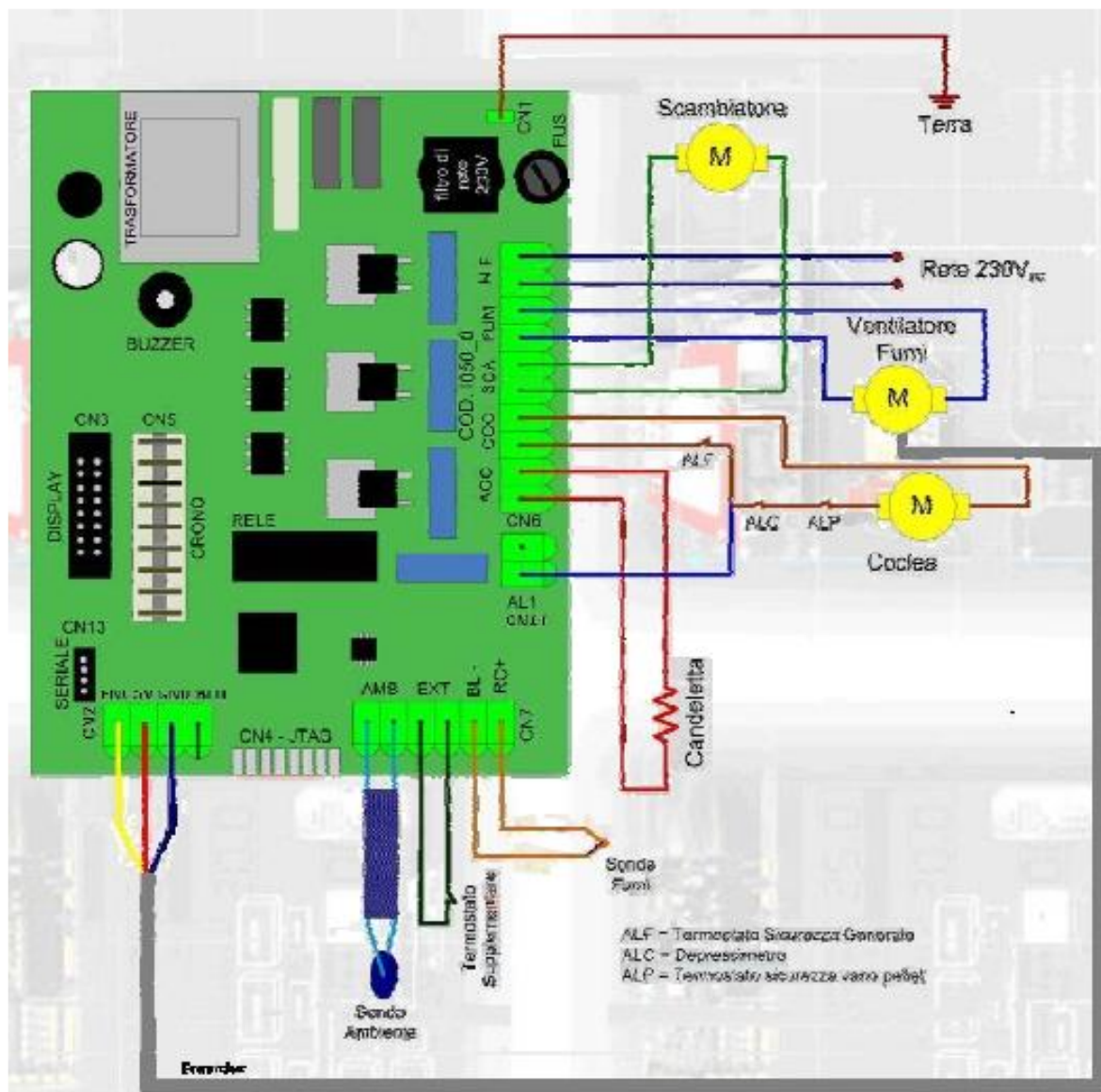
Slika 9.17. Elektronska kartica
