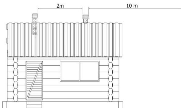
Slika 5.9a - Dimnjak - pozicioniranje i udaljenost
